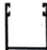
GUIDA ALLUMINIO 30x24x30
